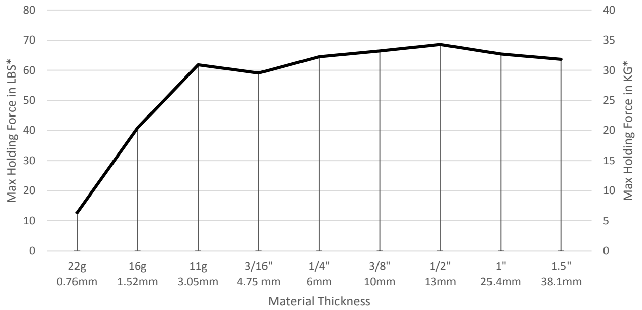
Magswitch Mini Multi Angle Breakaway Data vs. Thickness
